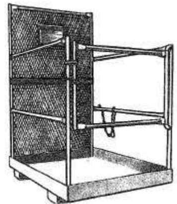
Una plataforma de trabajo para montacargas tiene barandas regulares y una rejilla para impedir contacto con las partes movientes del mástil. Una cadena asegura la plataforma al mástil.
