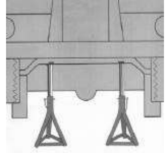
Torres de soporte (jack stands) colocadas debajo del vehículo después de ser levantado con un gato.
