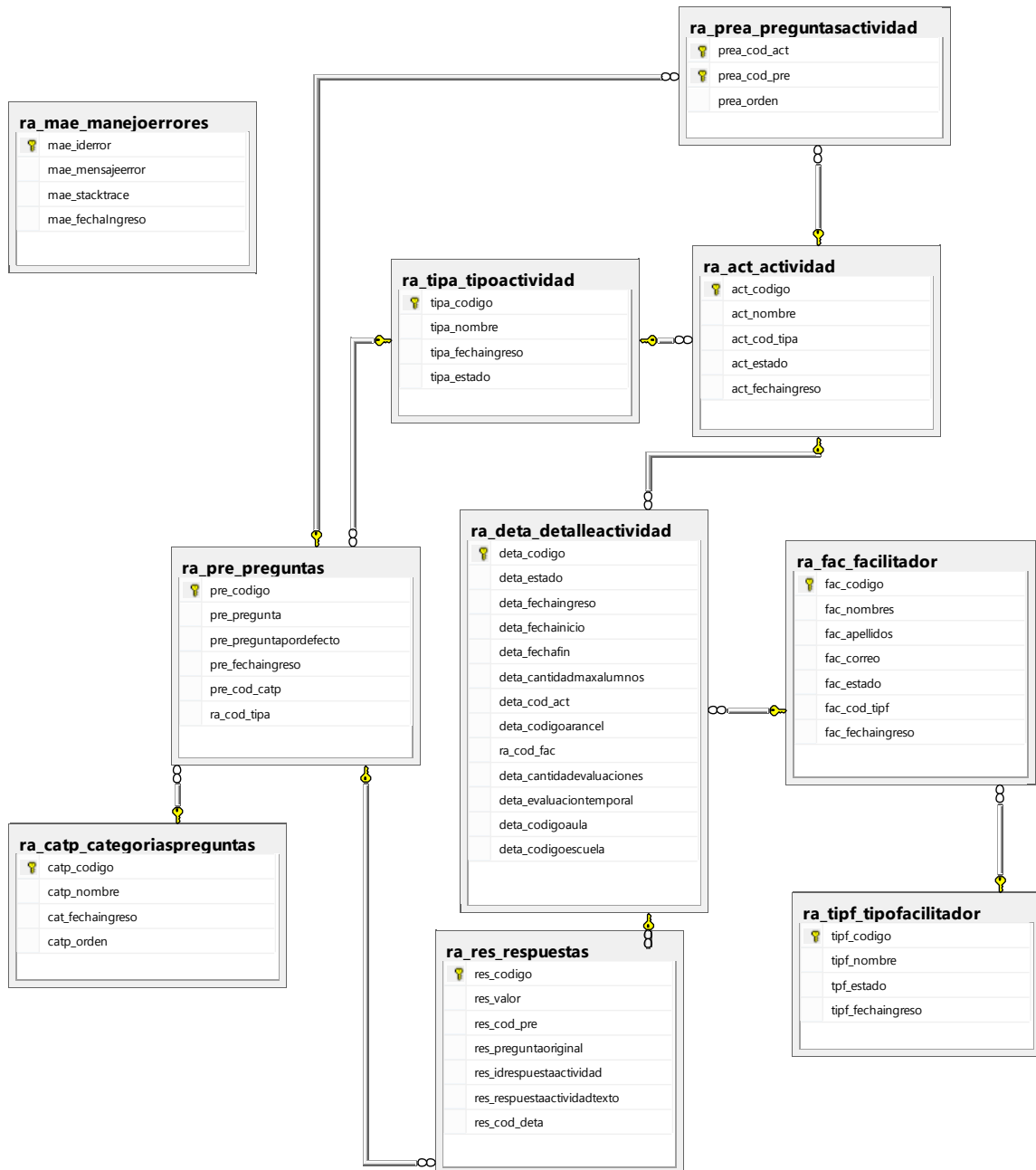
Ilustración 4. Diagrama de base de datos. Elaboración Propia
