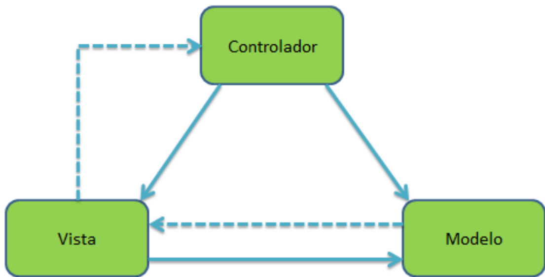
Ilustracion 3 Representacion Grafica del Modelo Vista Controlado.
