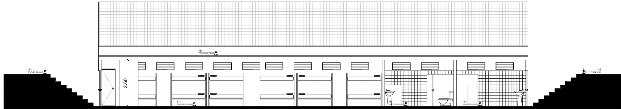
PLAZA ZURITA SECCIÓN C-C SIN ESCALA
