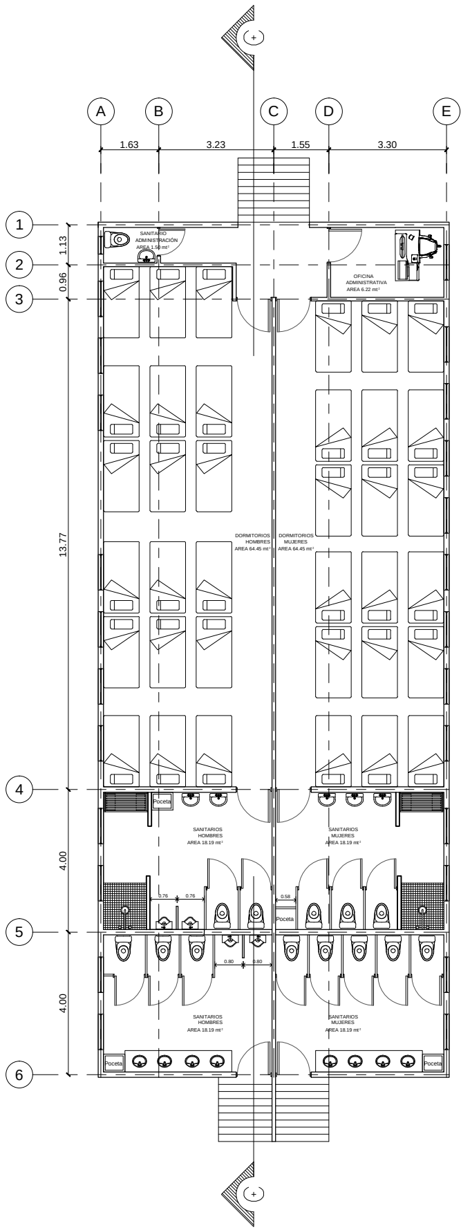
PLANTA ARQUITECTONICA - DORMITORIOS Y SANITARIOS PLAZA ZURITA SIN ESCALA
