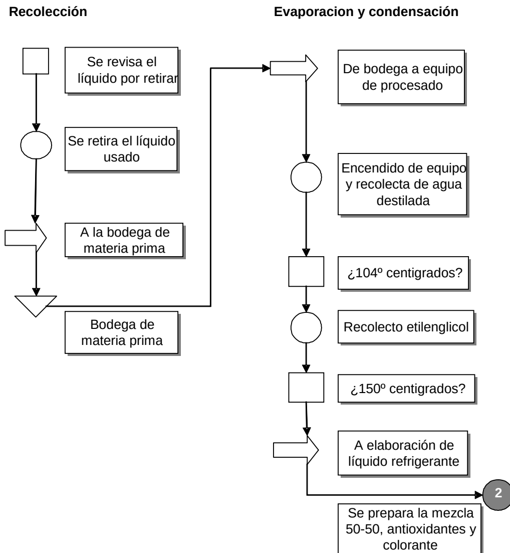
Figura No. 14 Diagrama de flujo del proceso productivo de la planta de reciclaje.
