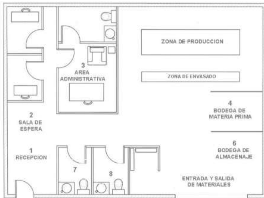
Figura No. 16 Diseño propuesto de distribución en planta.
