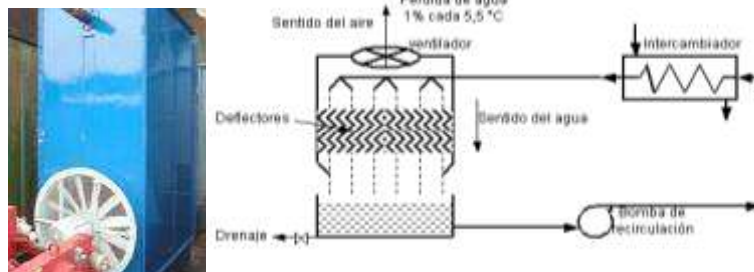
Figura No. 20. Torre de enfriamiento de agua y diagrama de un sistema de enfriamiento por aire.
