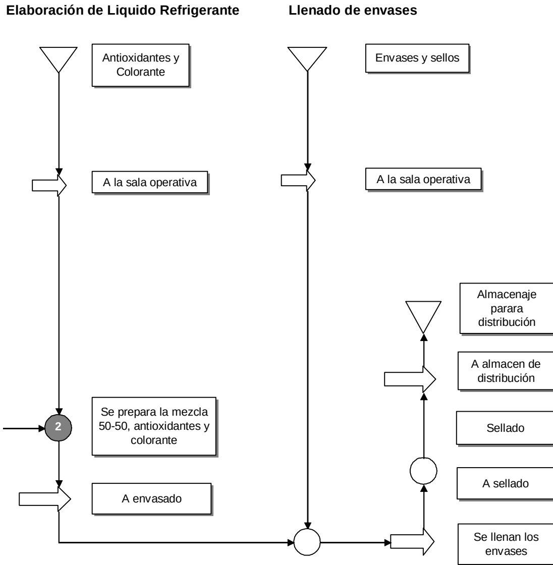
Figura No. 15 Diagrama de flujo del proceso productivo de la planta de reciclaje.
