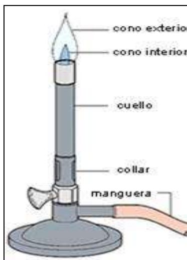
Figura. No. 19 Diagrama de un mechero de Bunsen.
