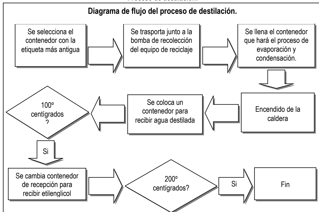
Figura No. 10 Proceso de destilación.
