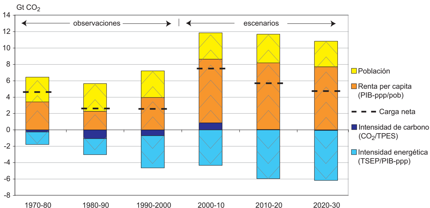
Gráfico RT.3: Descomposición de los cambios de las emisiones mundiales de \text{CO}_2 relativas a la energía a escala mundial para los tres decenios pasados y los tres decenios futuros [Gráfico 1.6].
