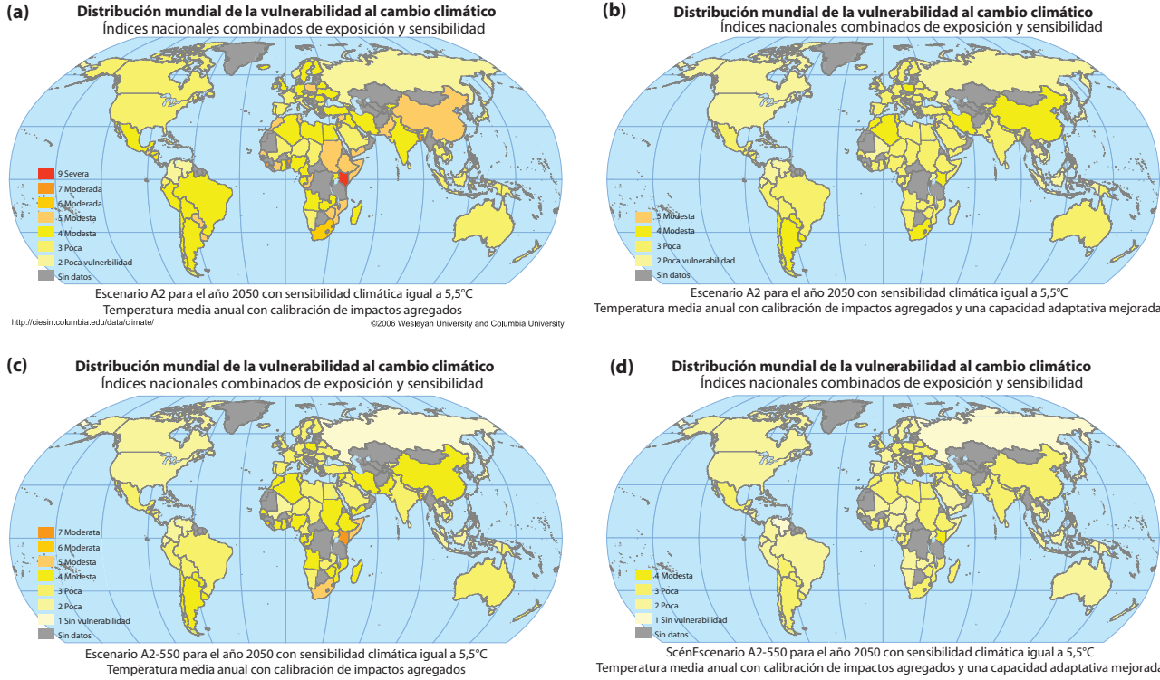
Figura RT.19. Distribuci n geogr fica de la vulnerabilidad en el a o 2050 con mitigaci n y sin ella, junto con un escenario de emisiones A2 del IE-EE, con una sensibilidad clim tica de 5.5 C. El Panel (a) describe la vulnerabilidad con una representaci n est tica de la capacidad adaptativa actual. El Panel (b) muestra la vulnerabilidad con una capacidad adaptativa mejorada mundial. El Panel (c) describe las implicaciones geogr ficas de la mitigaci n dise ada para contener las concentraciones efectivas de gases de efecto invernadero en la atm sfera a 550 ppm. El Panel (d) ofrece una descripci n de los efectos complementarios combinados de la mitigaci n al mismo l mite de concentraci n de 550 ppm y la capacidad adaptativa mejorada. [F20.6]
