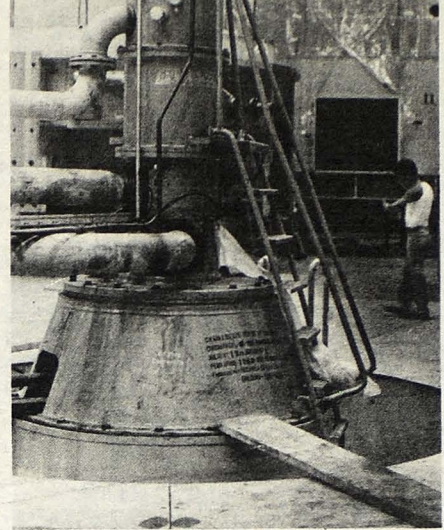
GENERADOR. Parte superior de la primera unidad generadora de San Lorenzo, con capacidad de 90 mil kilovatios, que emerge del profundo pozo donde ha sido montado el generador con la respectiva turbina de eje vertical. La obra la realiza el consorcio suizo-italiano COGEFAR-CSC.
