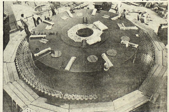
ROTOR GIGANTE. Rotor de la segunda unidad generadora de la Central Hidroeléctrica de San Lorenzo, captado en la etapa preparatoria de su montaje en la casa de
