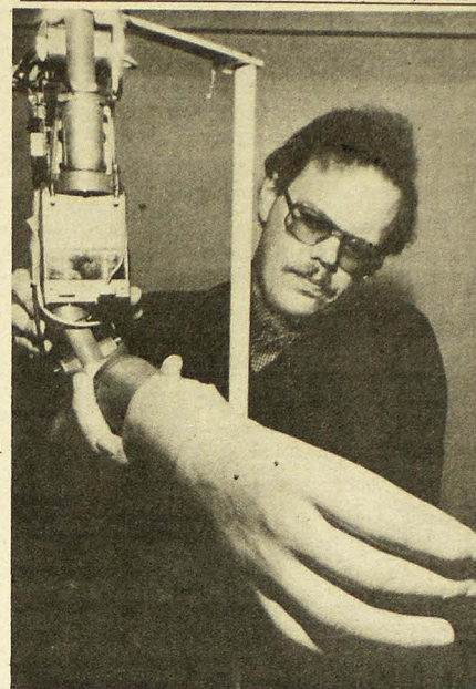
BRAZO HIDRAULICO. Hanóver, Alemania Occidental, julio (DaD). Un técnico especialista del Instituto de Mecánica, de la Universidad de Hanóver, muestra el "más completo" brazo ortopédico del mundo, que ha sido contruido por un equipo técnico de la universidad y que funciona hidráulicamente.
