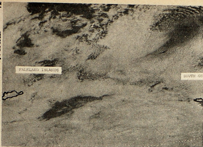
SATELITE FOTOGRAFIA LAS MALVINAS. — Washington, mayo 2. Fotografía de satélite muestra las condiciones del tiempo en las islas Malvinas, que están cubiertas de una espesa capa de nubes. Aparece también una parte de la costa argentina y las islas Georgias del Sur. (UNIFAX II de UPI).
