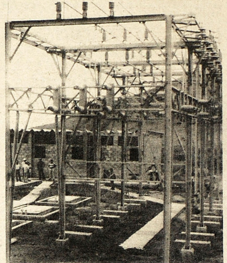
SUB ESTACION. En breve quedarán concluidos los trabajos de la Sub Estación Eléctrica que abastecerá energía a la Estación Central de Bombeo del Proyecto Zona Norte de ANDA, que mejorará a corto plazo el abastecimiento de agua potable en la zona metropolitana de San Salvador.
