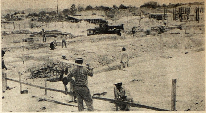
TERRACERIA. Fue concluida la terracería para los siete edificios de cinco plantas cada uno, que el Instituto de Vivienda Urbana construirá en el Centro Urbano Zaca-
